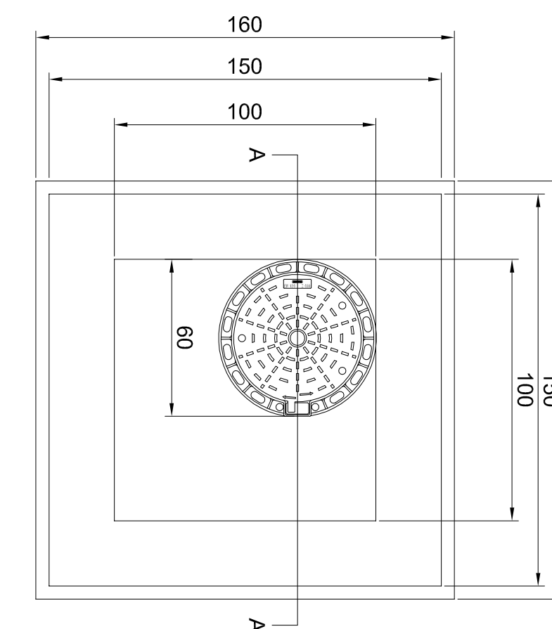
PIANTA POZZETTO B.T.
