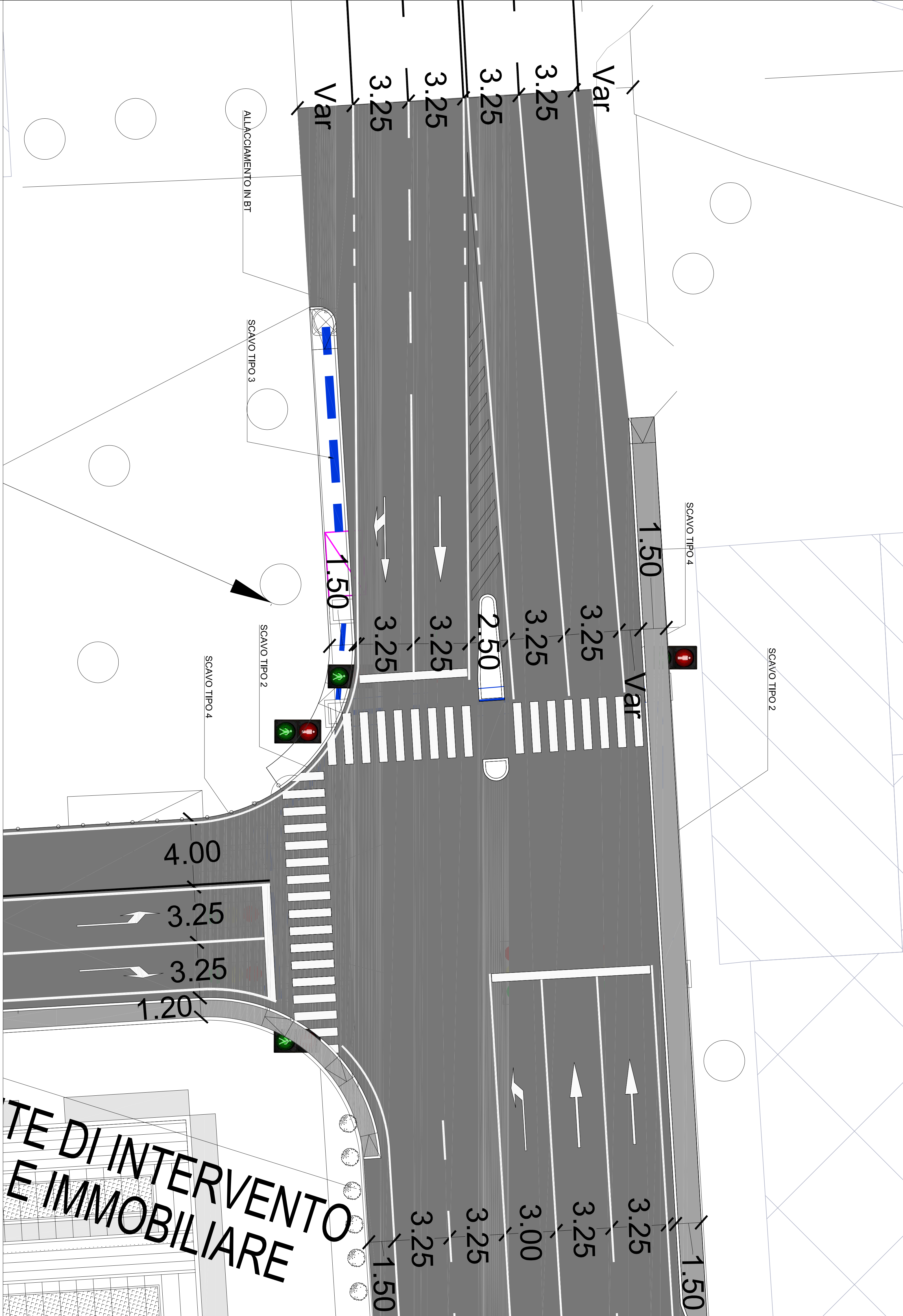
SCHEMA TIPICO IMPIANTO SEMAFORICO
